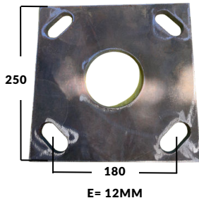
DETALLE DE LA PLACA
