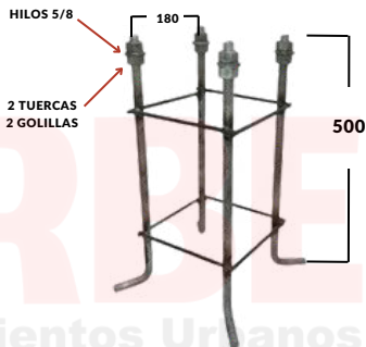
DETALLE DEL CANASTILLO
