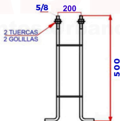
DETALLE PLACA BASE
