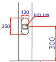
DETALLE TAPA DE REGISTRO
