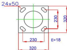
DETALLE PLACA BASE
